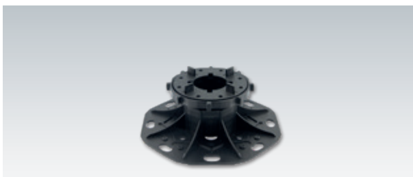
Terrassen-/Balkonstelzager fix inkl. Aufsatzstück (für Fugenbreite 3 mm)
