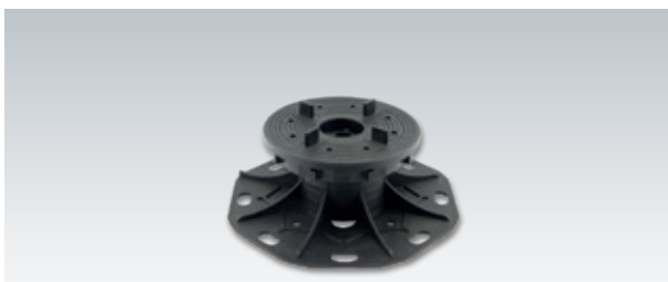
Terrassen-/Balkonstelzager selbstnivellierend inkl. Aufsatzstück (für Fugenbreite 3 mm)
