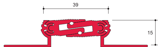
FAL 4015-DR
