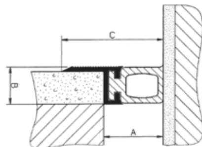
Sportbodenprofil als Wandanschluss
