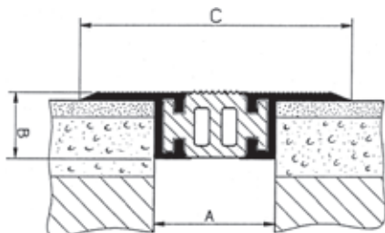
Sportbodenprofil
