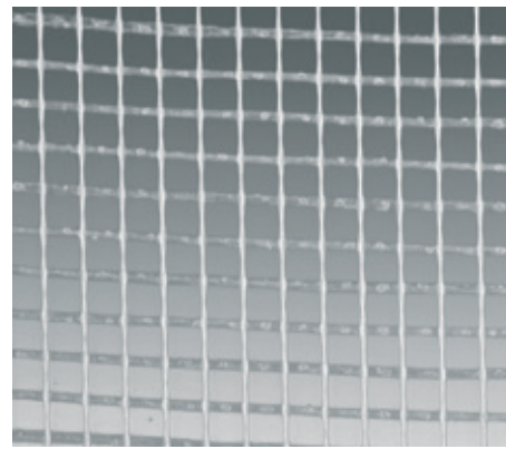
Glasgittergewebe FG 105, Maschenweite: 7 x 7 mm
